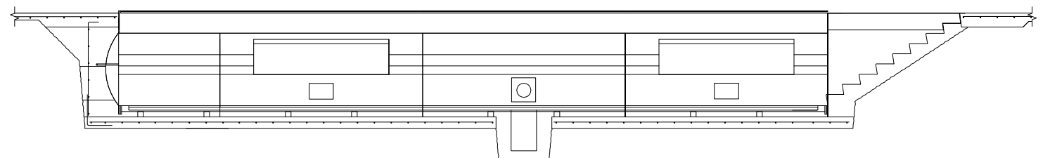
42' IN-LINE LONGITUDINAL SECTION \frac{1}{4}'' = 1'-0''
