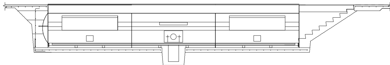
36' IN-LINE LONGITUDINAL SECTION \frac{1}{4}'' = 1'-0''
